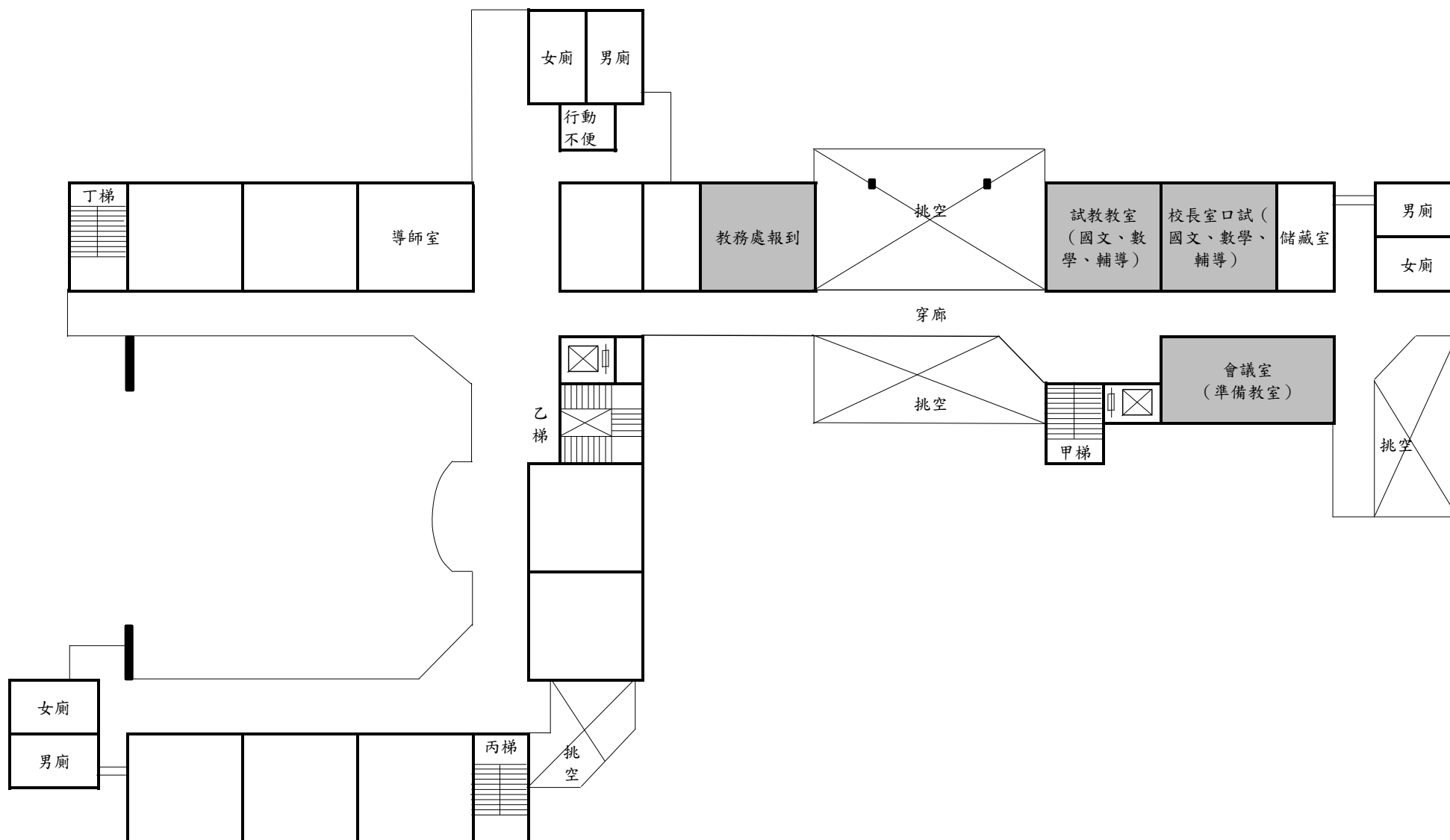
二樓平面圖
